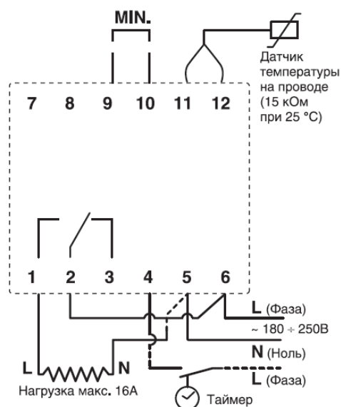
Рис.2. Схема подключения devireg™ 316 .
